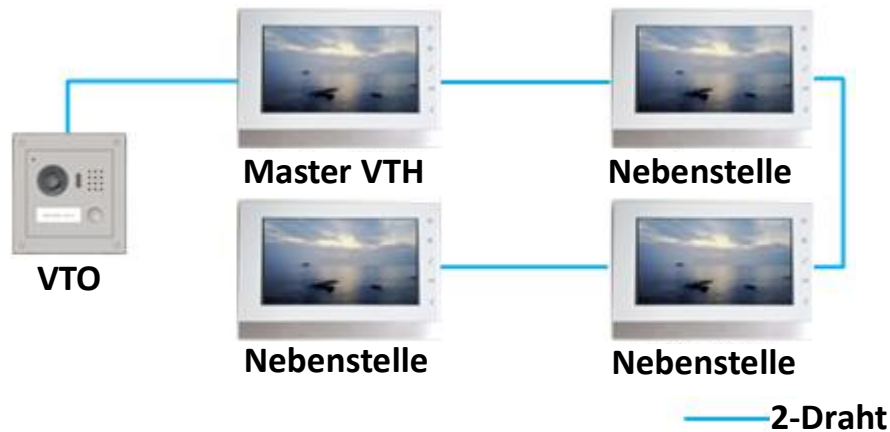
Abbildung 1–1 Einfamilienhaus-Netzwerk 1
