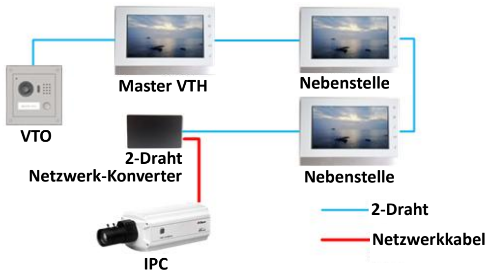
Abbildung 1–2 Einfamilienhaus-Netzwerk 2
